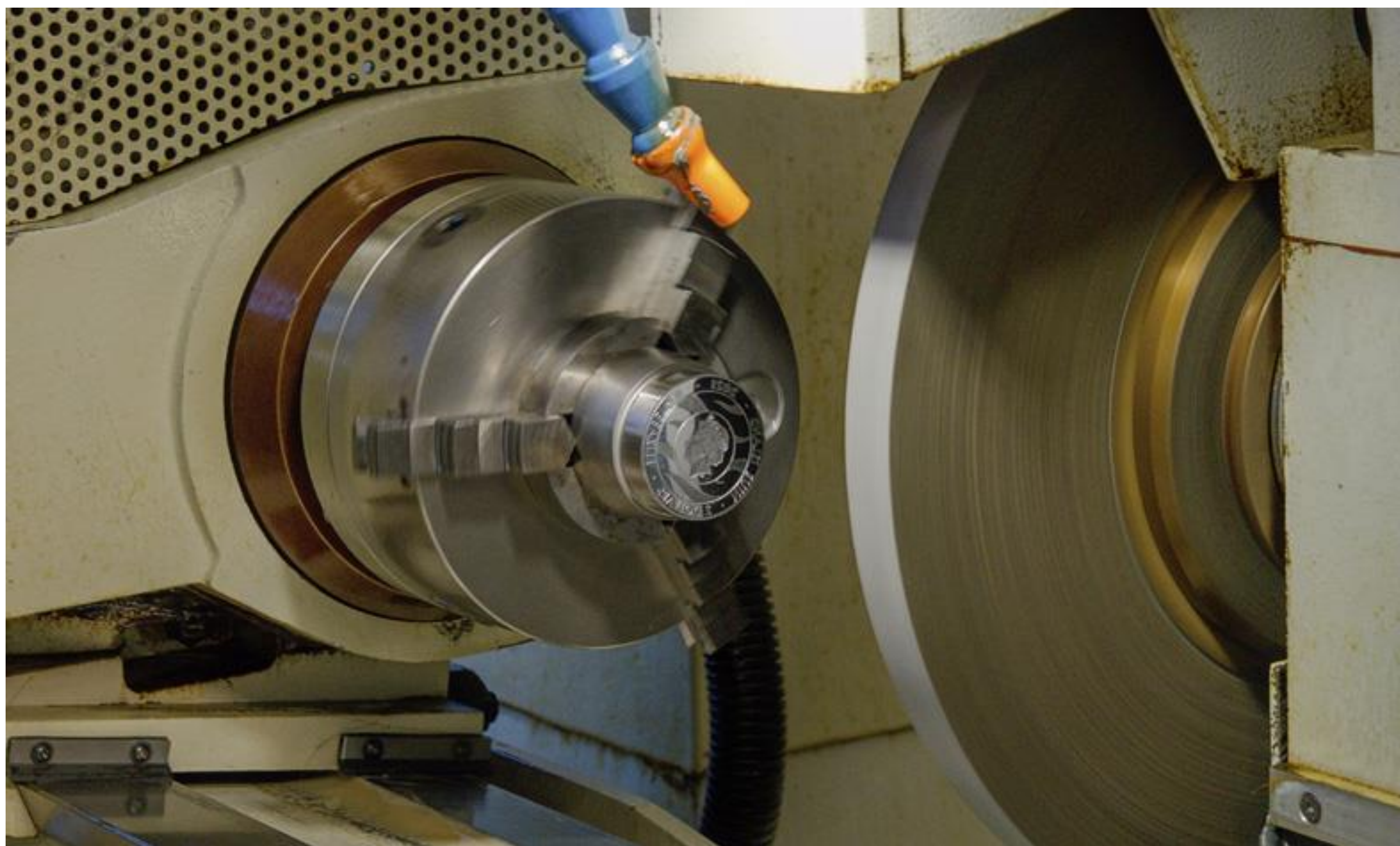
obrábění razidel do konečné geometrie
