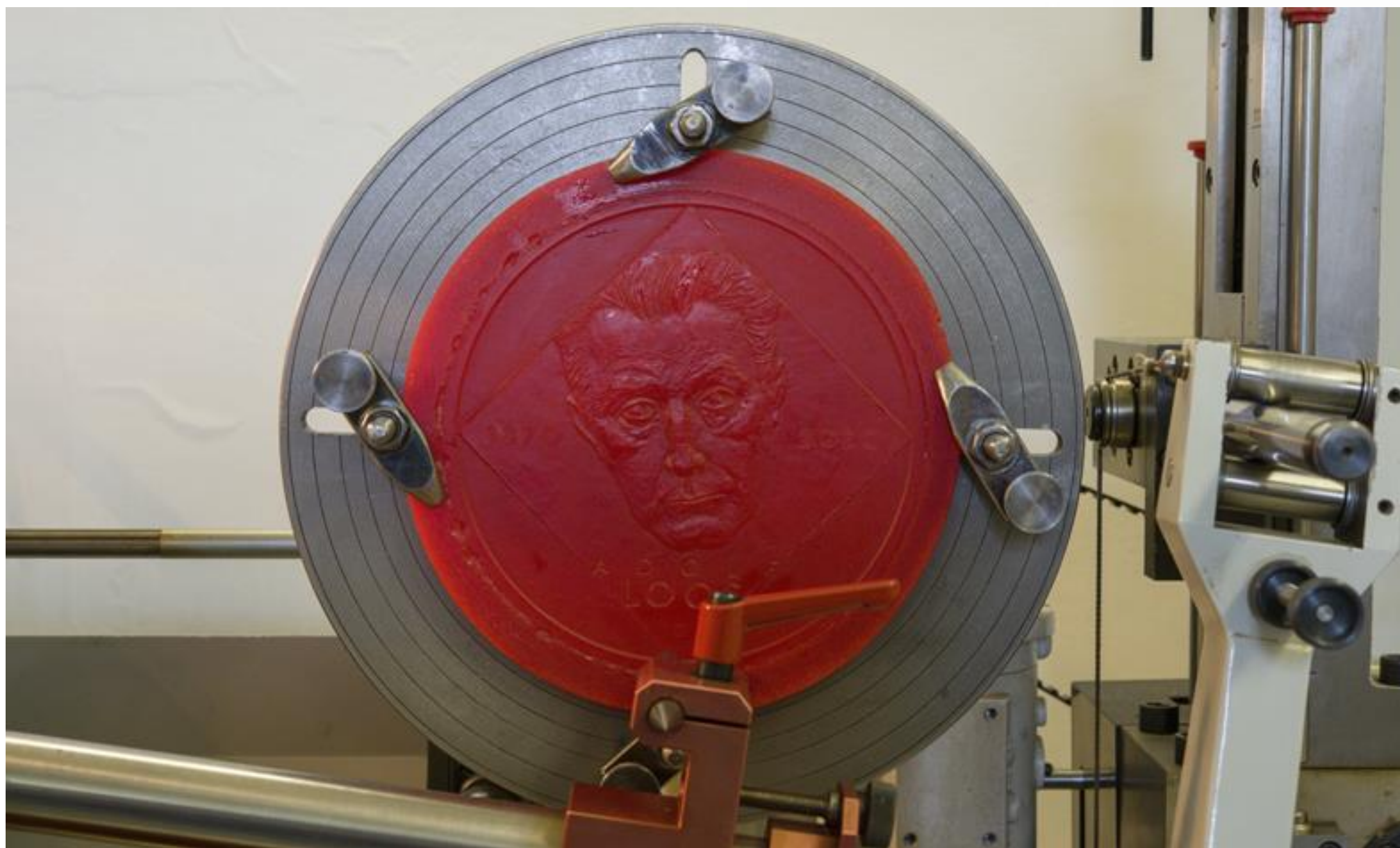
snímací agregát, redukováný pryskyřicový odlitek
