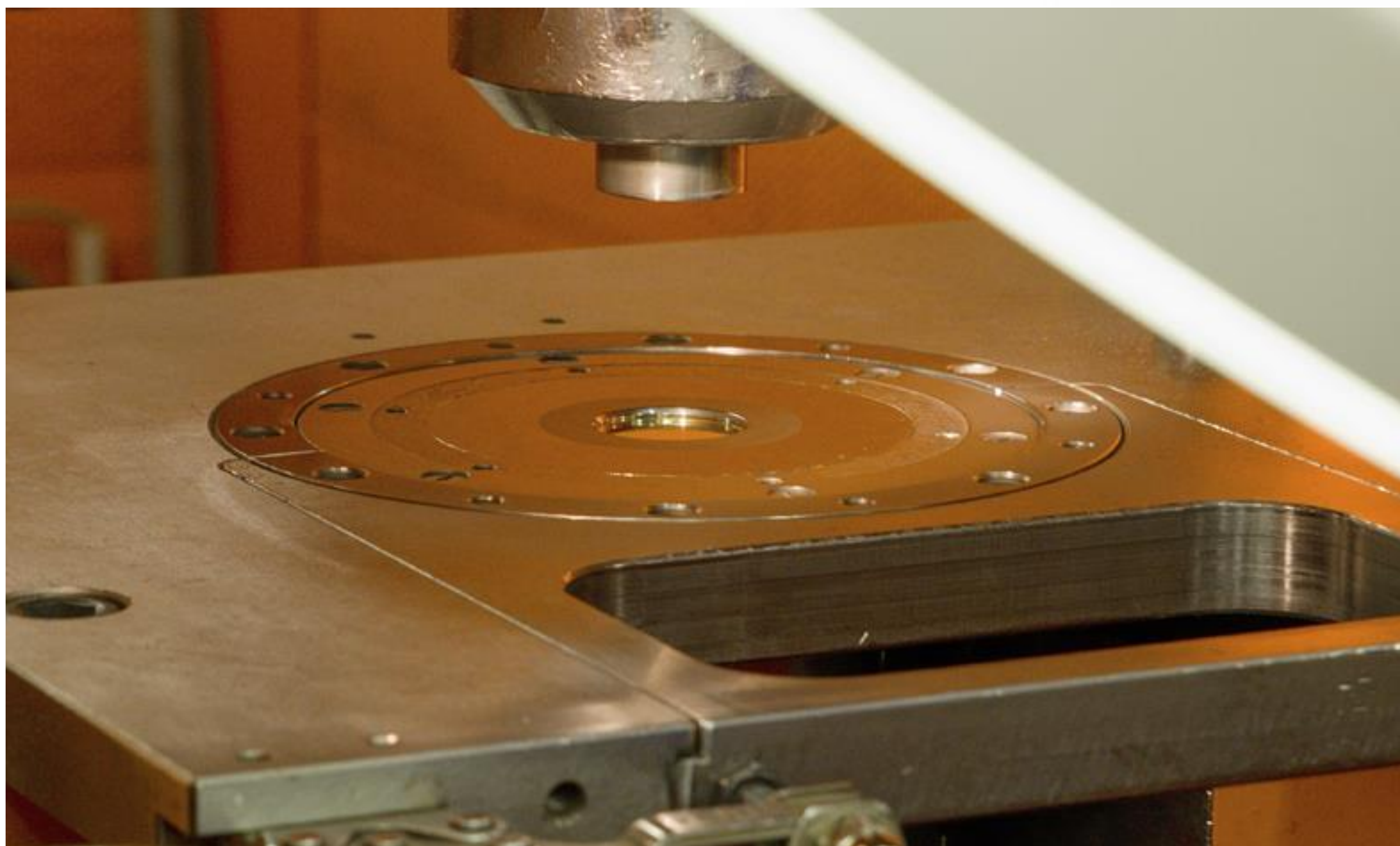
ražba (horní razidlo před zdvihem)
