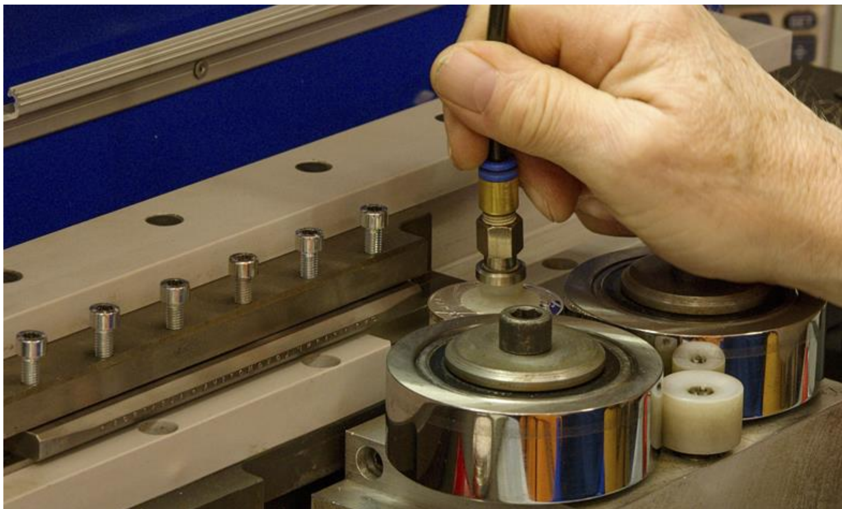
lisování nápisu na hraně
