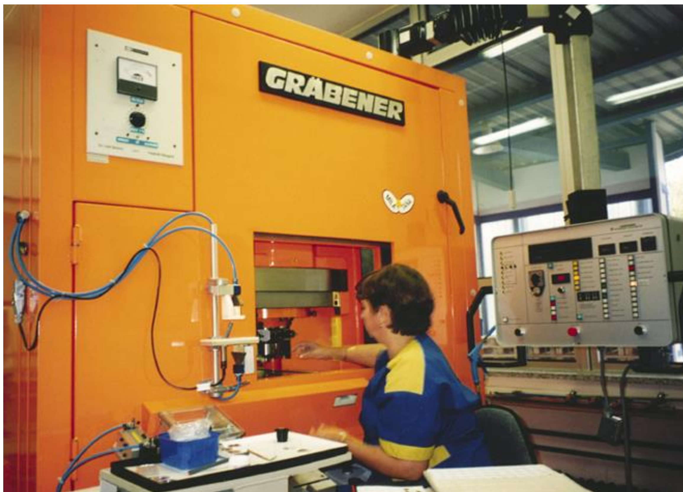
ražba na lisu Gräbener
